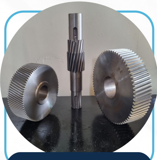
Engrenagens e eixo pinhão helicoidal
